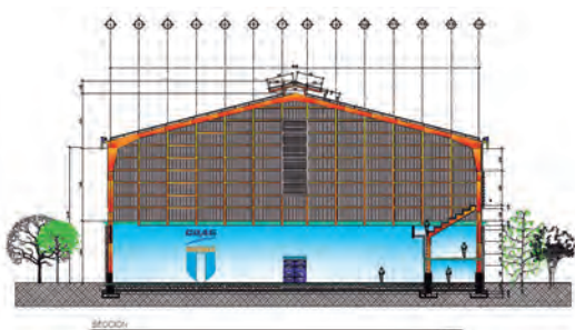
Plano de sección transversal Interior graderíos, áreas de vestidores, servicios y oficinas
