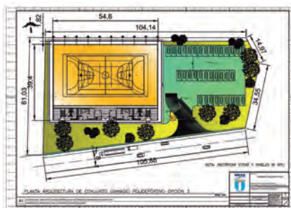
Plano de conjunto Planta de Arquitectura del Gimnasio Polideportivo San Juan Gascón Sacatepéquez
