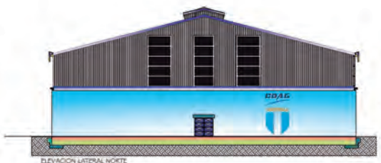
Elevación lateral Norte del Pabellón Deportivo para la práctica de baloncesto Chimaltenango
