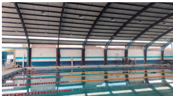
Reparación de cubierta de la piscina del Complejo Deportivo de Quetzaltenango
