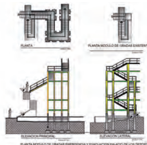
Plano de Elevación propuesta lado Norte del módulo de gradas de Emergencia y Evacuación
